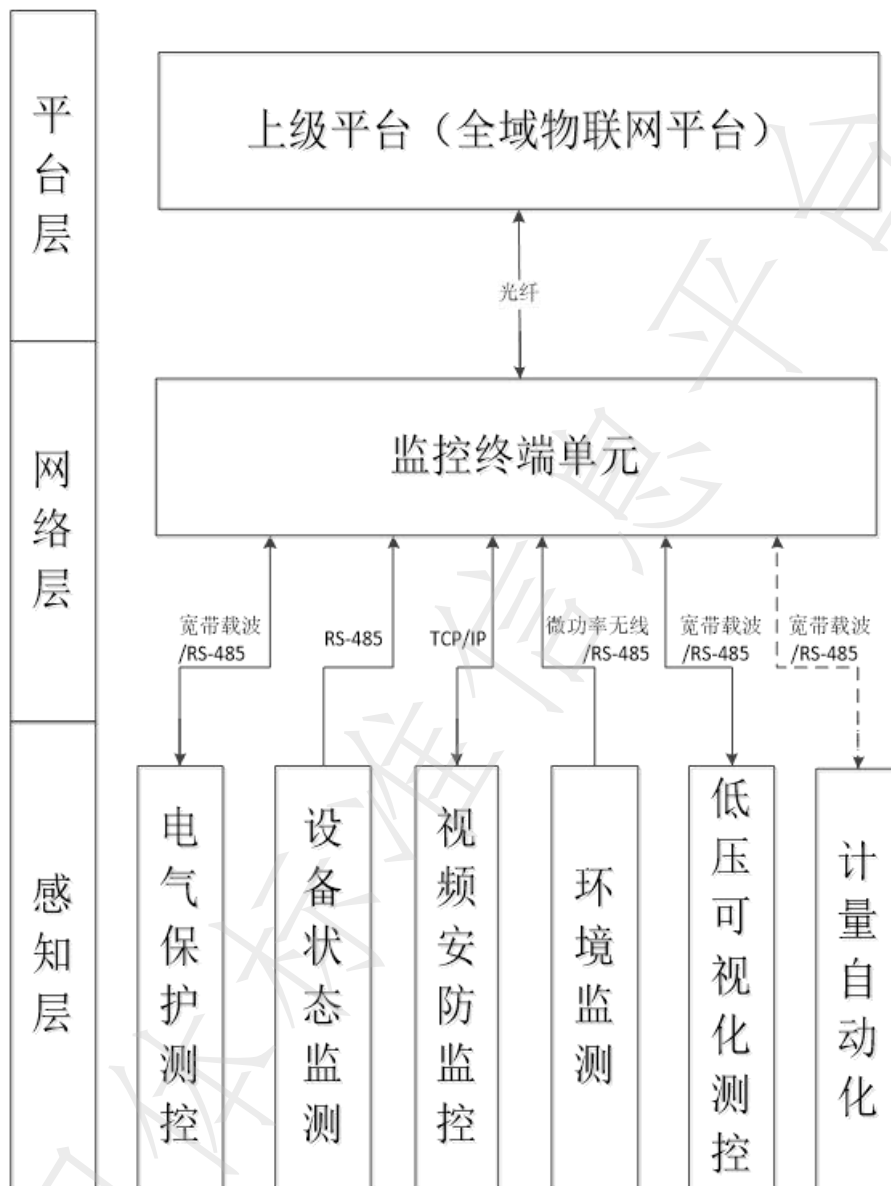
图2 智能配电站网络系统架构图
