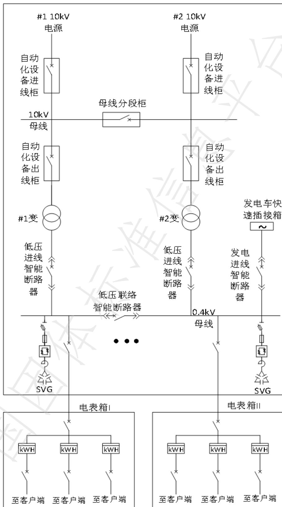
图1 智能配电站一次系统拓扑图
